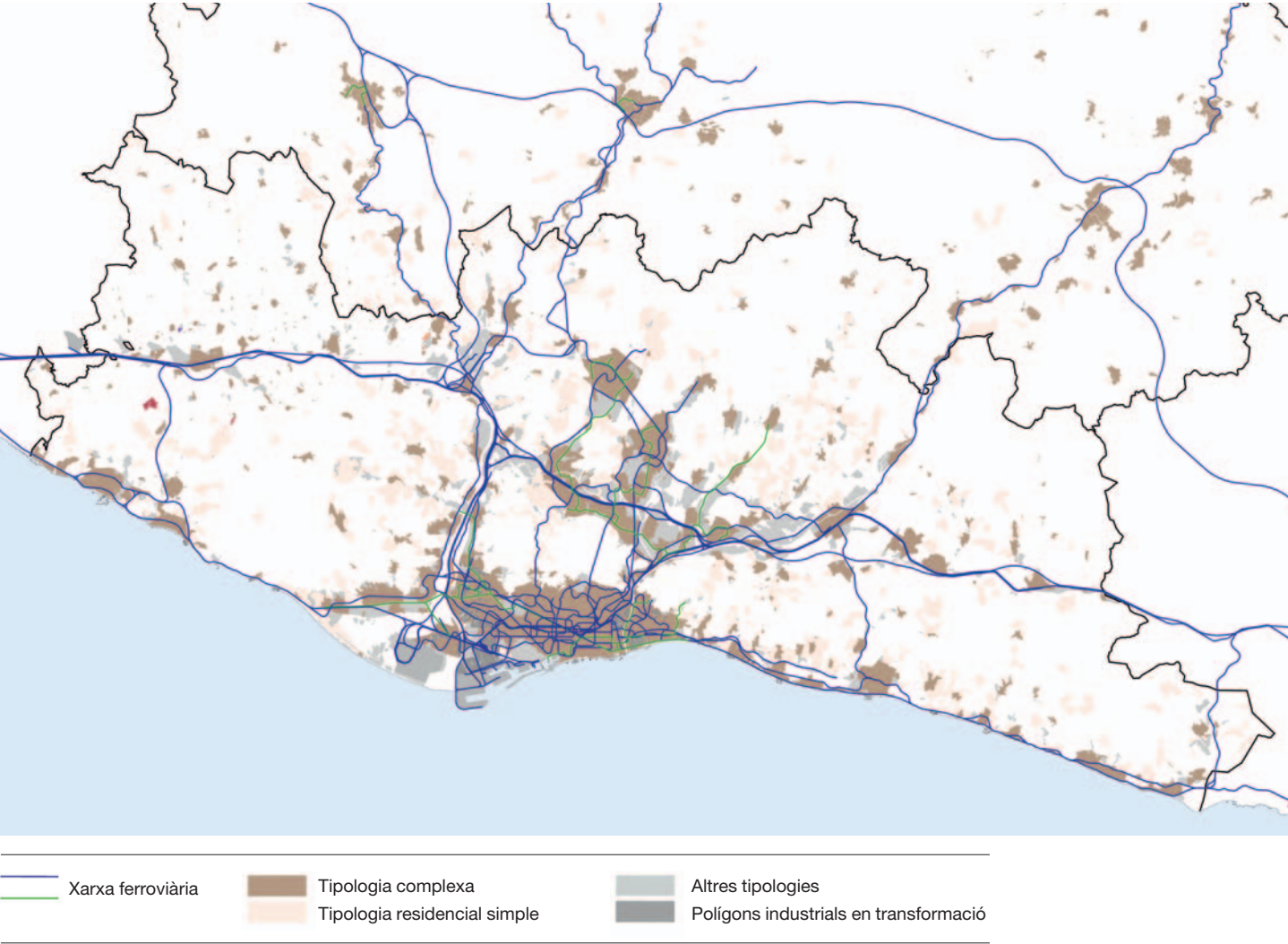
Mapa 7.67 El futur sistema nodal: la ciutat compacta i complexa i la seva relació amb la xarxa ferroviària
