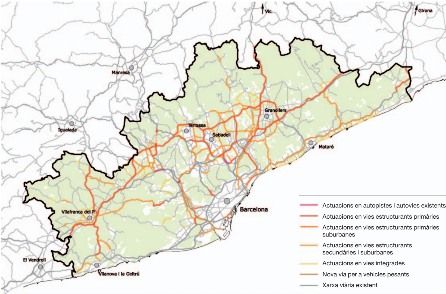
Mapa 7.45 Xarxa viària proposada
